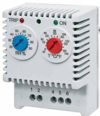
Exemple thermo-higrostat
