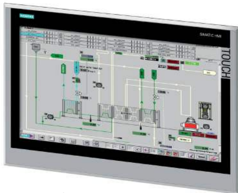
Ejemplo pantalla HMI 19"
