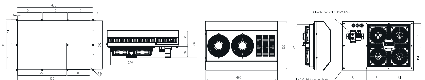
MVTEC300_230VF avec carcasse
