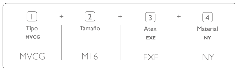
REFERENCIAS PRENSAESTOPAS POLIAMIDA EX/E
