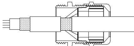
RÉFÉRENCES PRESSE-ÉTOUPES CEM MÉTRIQUE LAITON NICKELÉ
